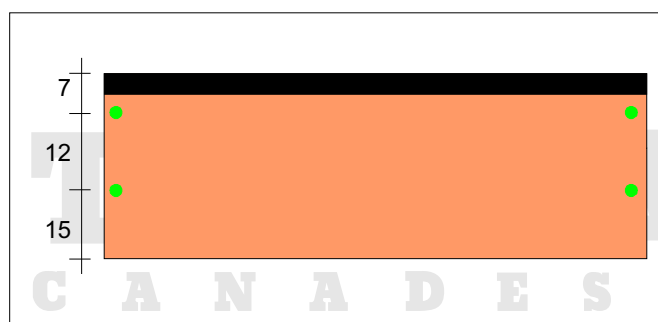
Fig. 5 - Chiodatura della prima fila di tegole
