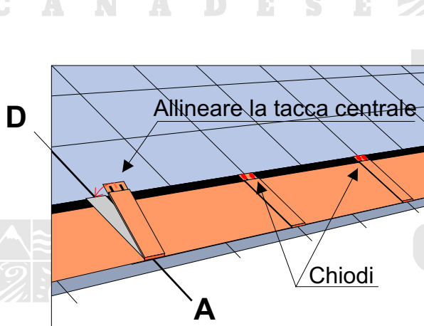
Fig. 8 - Applicazione del Compact Clip
