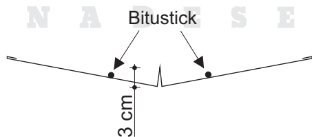
Fig. 15 - Compluvio indicativo
